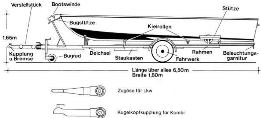
Anhänger 2-Rad für Mehrzweckboot (Trailer)
