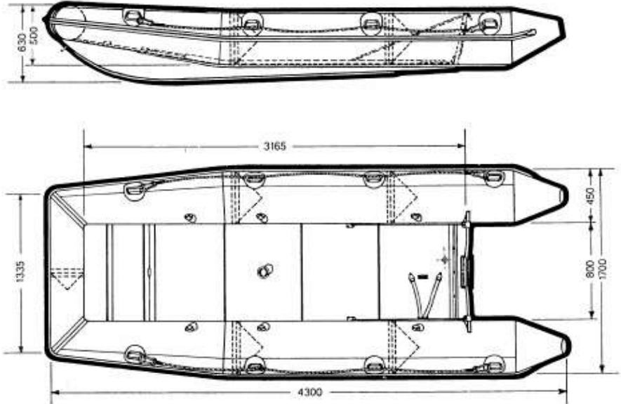
Schlauchboot Typ 430/170 ZEPHYR
